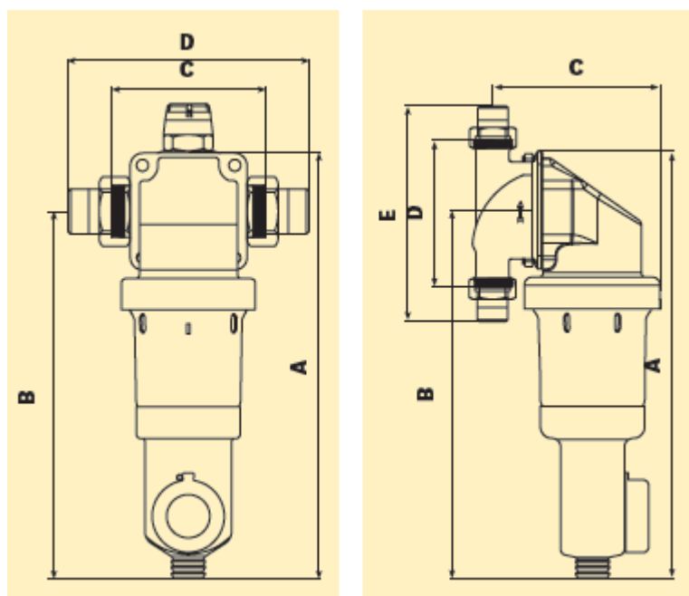
Filter brez reduktorja
